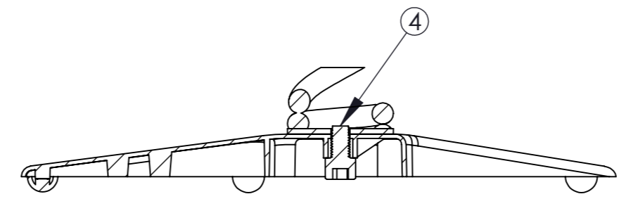
SECTION D-D SCALE 1 : 5
